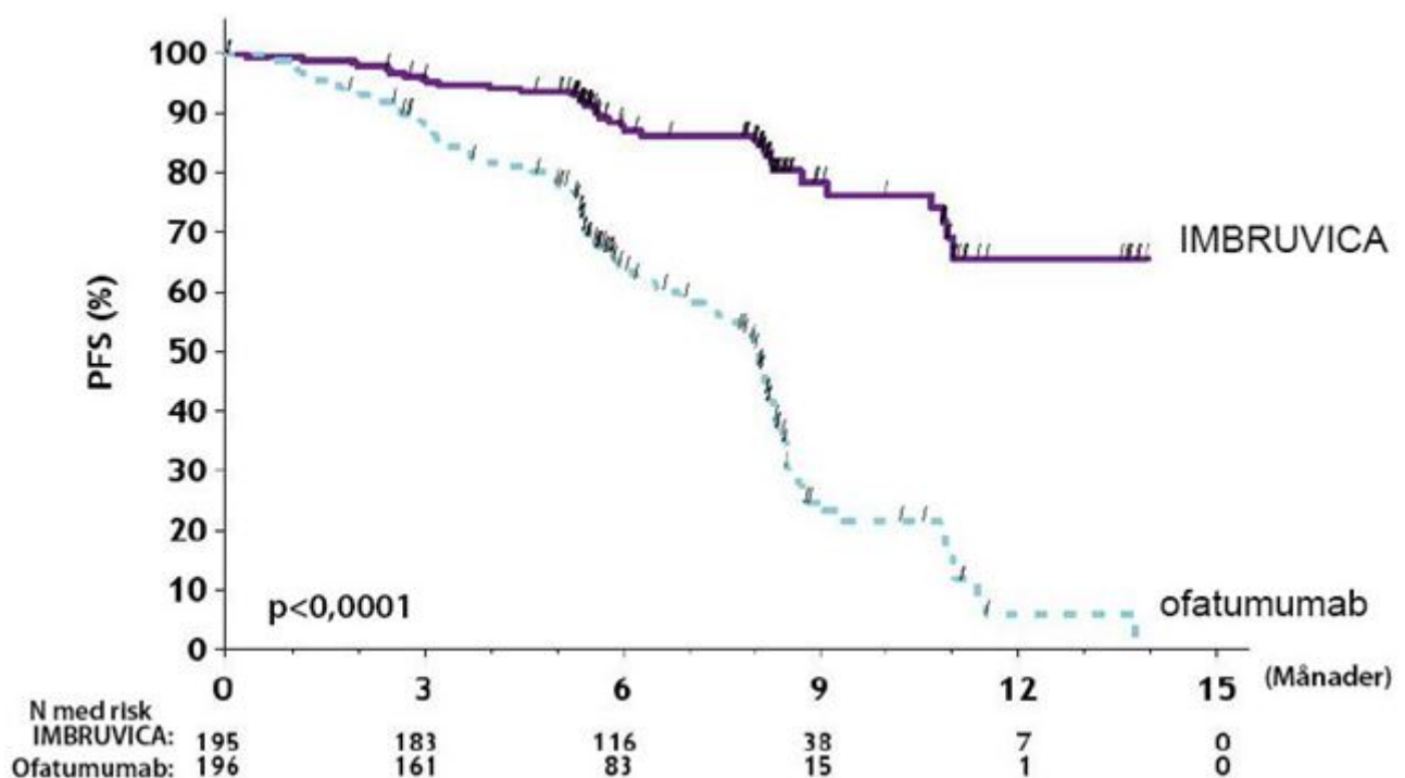
Figur 6: Kaplan-Meier-kurva för PFS (ITT-population) i studie PCYC-1112-CA
