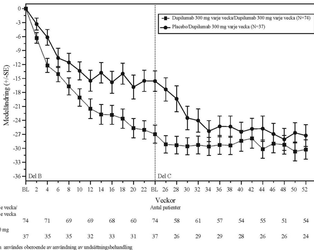
Figur 10: Medelförändring i DSQ-poäng från baslinjen över tid hos patienter i åldern 12 år och äldre med eosinofil esofagit (TREET del B och C)
