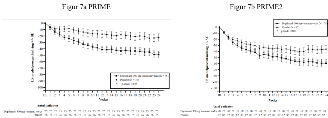
Figur 7. LS medelprocentändring från baslinjen i WI-NRS i PRIME och PRIME2 upp till vecka 24
