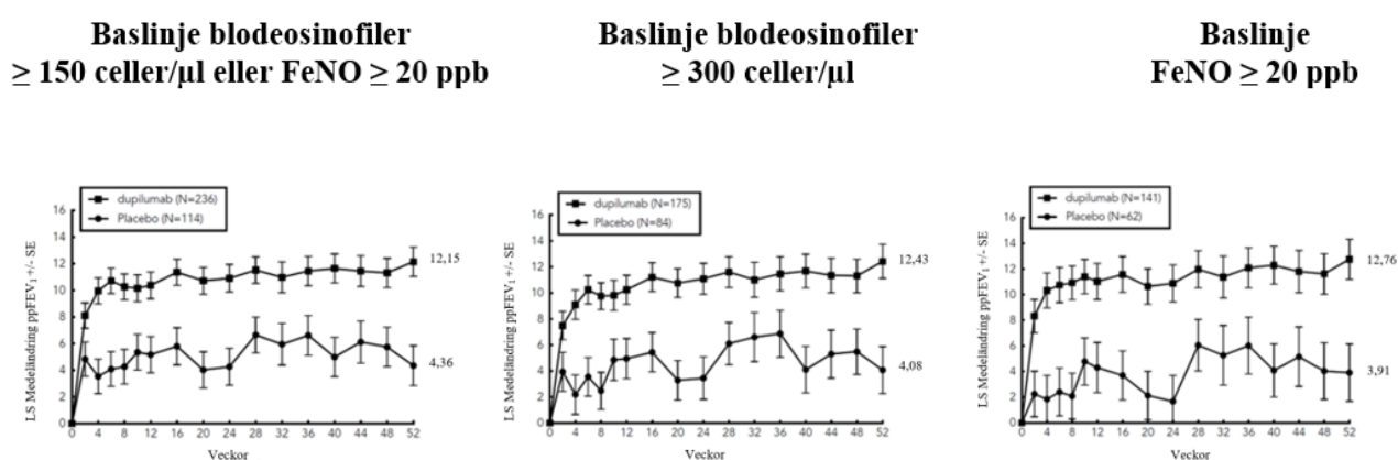
Figur 4: Genomsnittlig procentuell ändring från baslinjen av förväntad pre-bronkodilator FEV 1 (liter) över tid i VOYAGE (baslinje blod eosinofiler ≥ 150 celler/μl eller FeNO ≥ 20 ppb, baslinje eosinofili ≥ 300 celler/μl, och baslinje FeNO ≥ 20 ppb)
