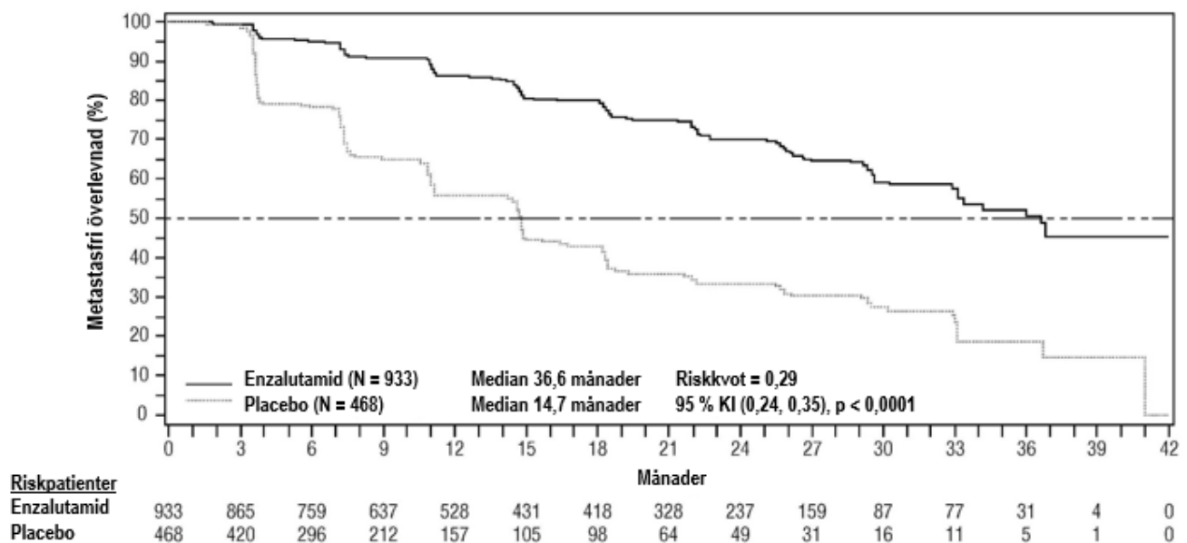
Figur 5: Kaplan-Meier-kurvor för metastasfri överlevnad i PROSPER-studien (intent-to-treat-analys)
